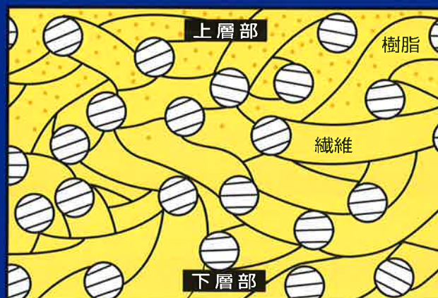
〈マリエース スーパーL 断面図〉
